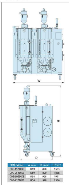
外形尺寸图 Dimensions
